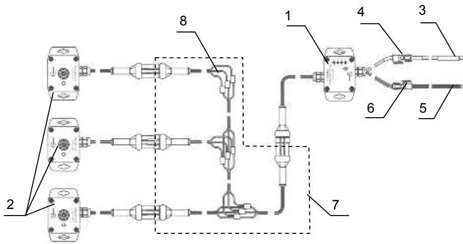
Рисунок 1 – Схема соединений блоков Системы
